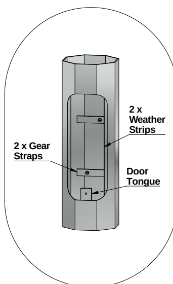
DOOR DETAIL
